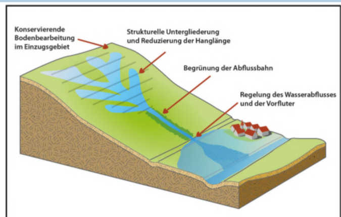
Abb. 3: Schematische Darstellung des Zusammenhanges zwischen der Abflussbildung auf Kulturlandflächen und den Möglichkeiten für abflusshemmende Maßnahmen zur Wasserrückhaltung. Quelle: INFRASTRUKTUR & UMWELT Prof. Böhm u. Prtn.
